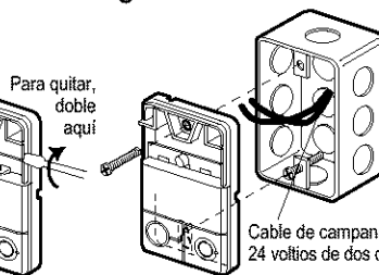
Figura 2 INSTALACIÓN PRE-CABLEADA
