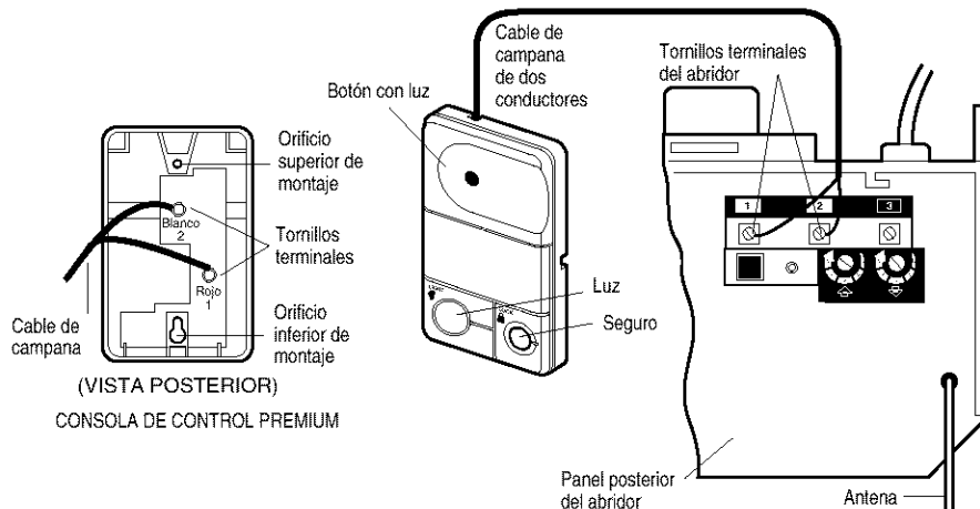
Cable de campana de 24 voltios de dos conductores en la caja múltiple
