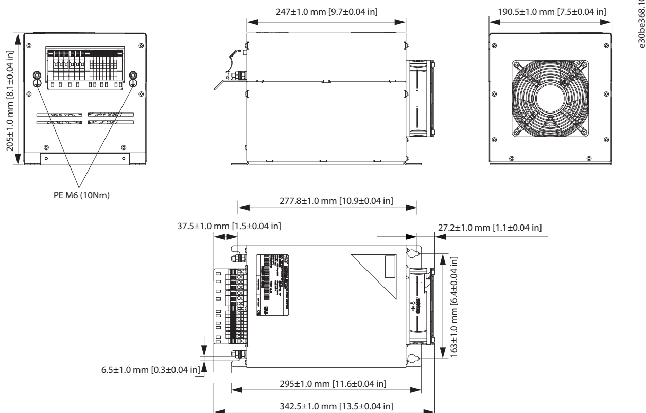
Illustration 7.4 IP20 X1-V3 External Fan
