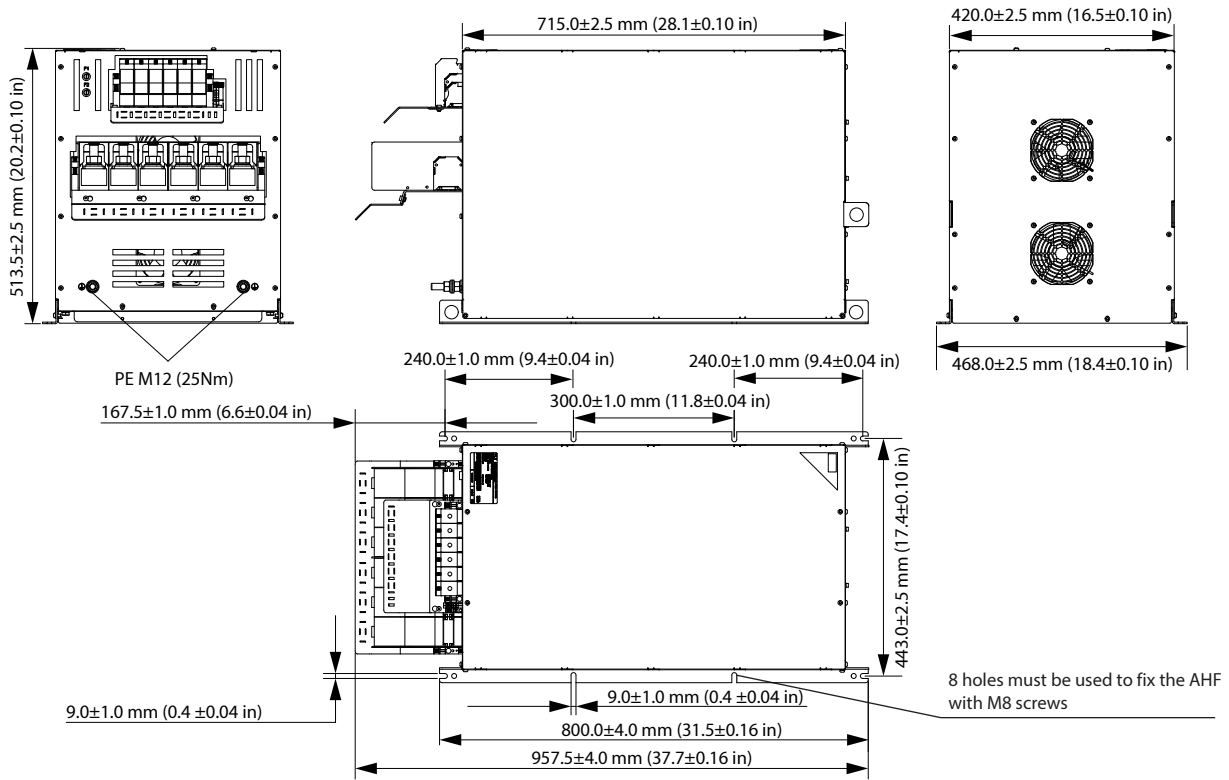
Figure 59: IP20 X8-V3 Internal Fan
