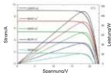
P-V-Kurven des PV-Moduls (120 W)
