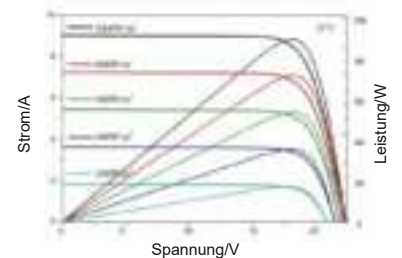
P-V-Kurven des PV-Moduls (100W)
