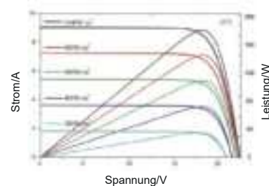
P-V-Kurven des PV-Moduls (195 W)
