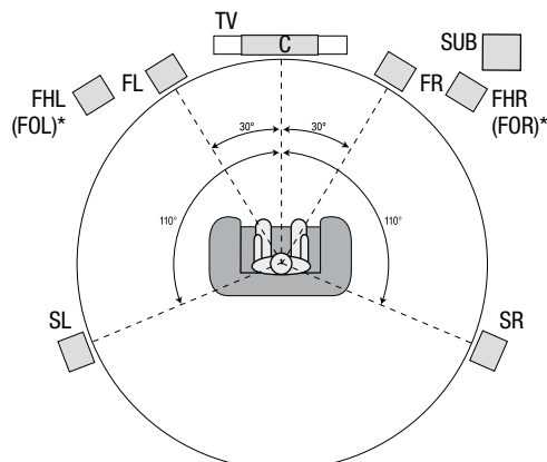
Lautsprecherpositionierung für 7.1-Kanal-Systeme (nur AVR 1710S/AVR 171S) (Mitte: mit rückwärtigen Surround-Lautsprechern. Unten: mit oberen Front-Lautsprechern)
