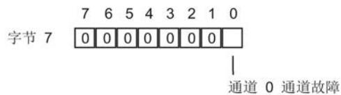
图 A-8 PM-E F pp DC24V PROFIsafe 诊断数据的第 7 个字节
