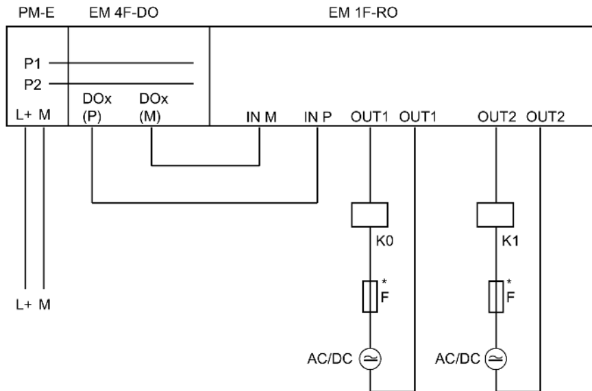
图 7-57 EM 1 F-RO DC24V/AC24..230V/5A 的接线图
