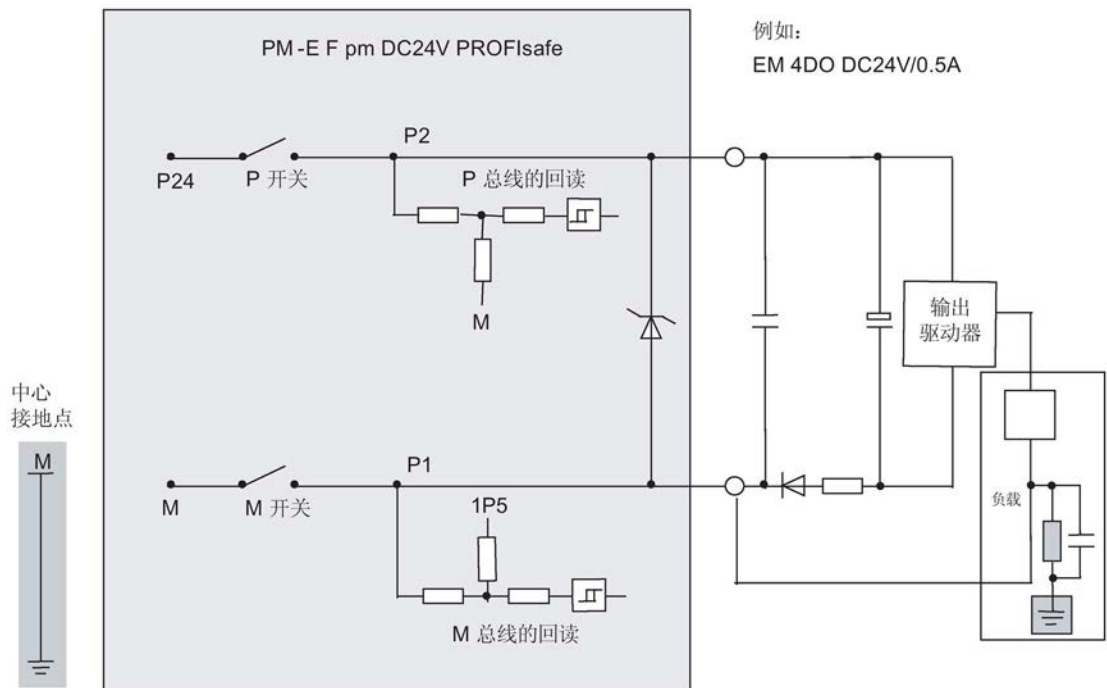
图 7-2 切换接地负载（机壳和接地之间存在电阻）
