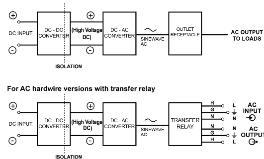
Abb. 5. Funktionsweise
