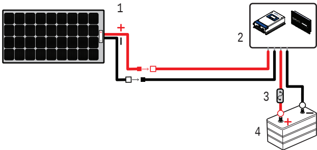
Figure 1 Schéma du câblage
